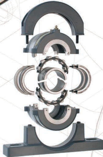
Palier à semelle en 2 parties type «Cooper»
