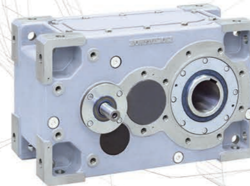
Une gamme complémentaire de réducteurs de très grosses capacités jusqu'à 400 Kw
